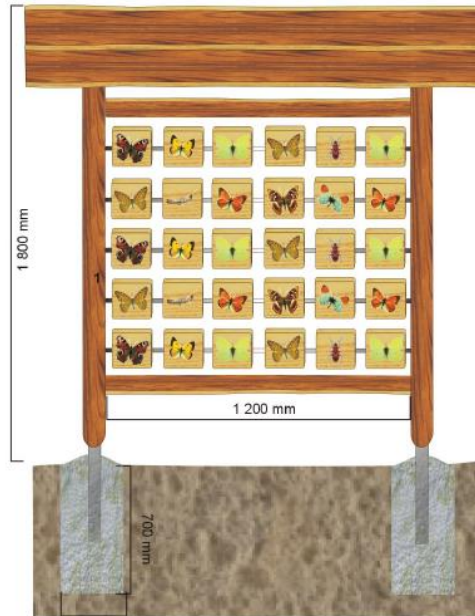
Pohled přední poměr 1:20
