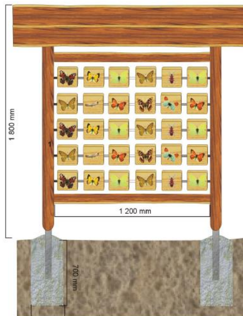
Pohled přední poměr 1:20
